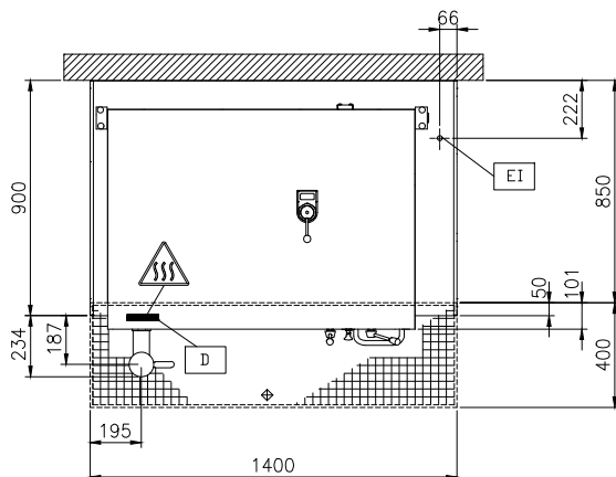
Boven aanzicht
